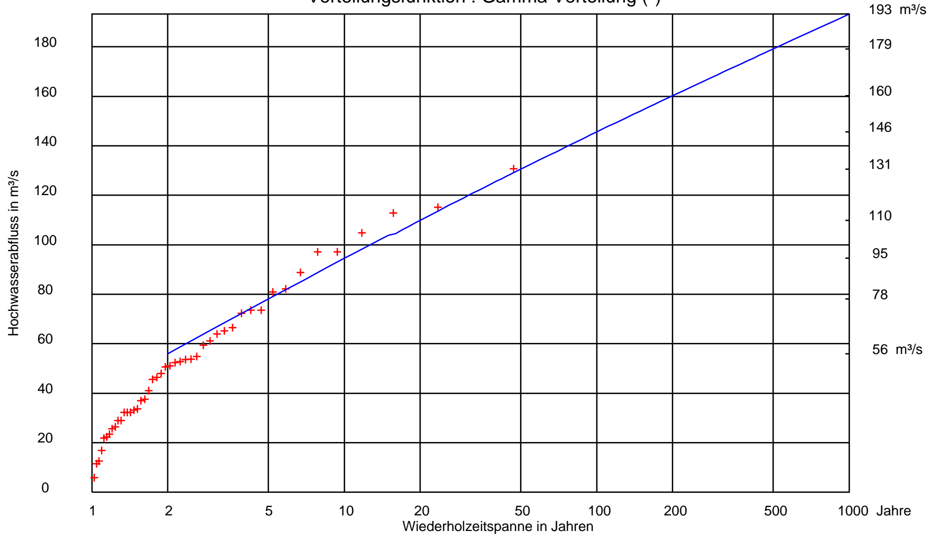
Verteilungsfunktion : Gamma Verteilung (*)
